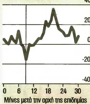
SARS (Χονγκ Κονγκ, 2002)
