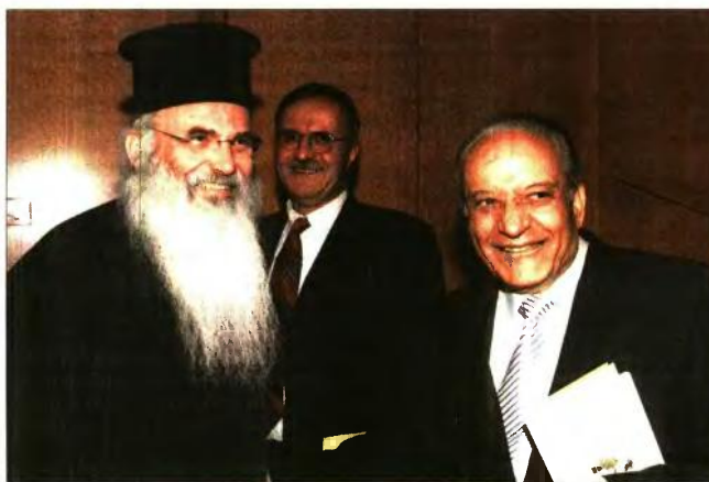
Με τον Μητροπολίτη Μεσοχώρας και Λαυρεωτικής κ. Νικόλαο. Πίσω του διακρίνεται ο αιμνηστος καθηγητής Ιατρικής Αστέριος Κασσαμούρης
